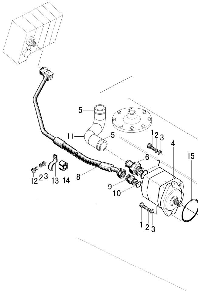
图 2 油泵总成 Fig. 2 Oil pump assy
