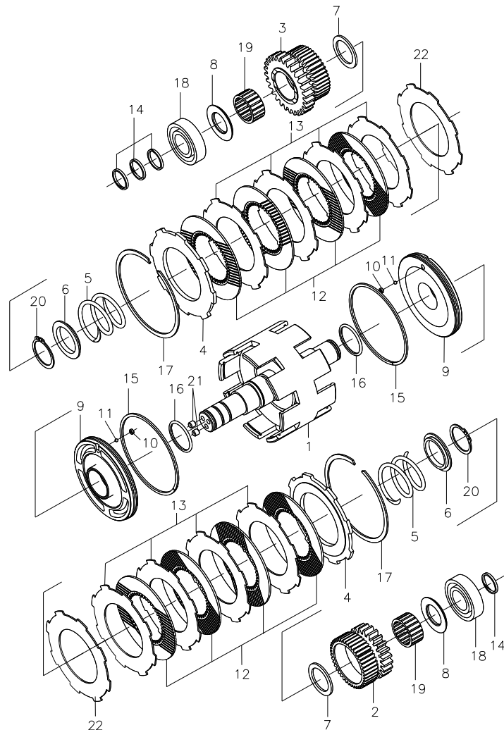
图 18 液力离合器(液力式) 中南 ZhongNan Fig.18 Hydraulic clutch(tor-con type)
