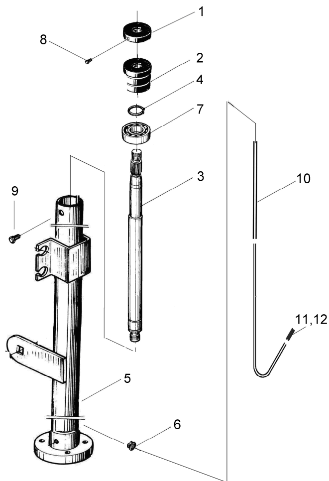
图2 转向管装置 Fig.2 Steering pipe device
