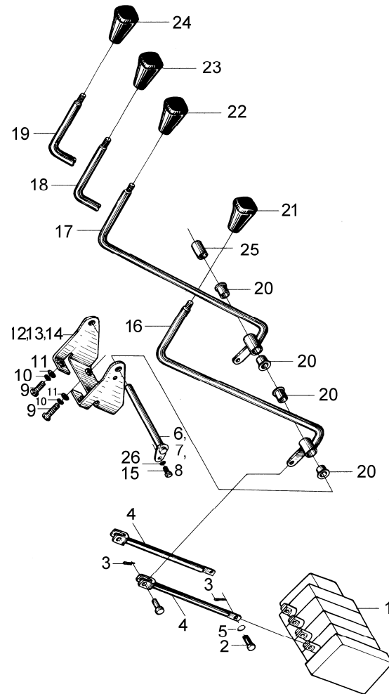
图 7 多路阀操纵 Fig.7 Multi-way valve control
