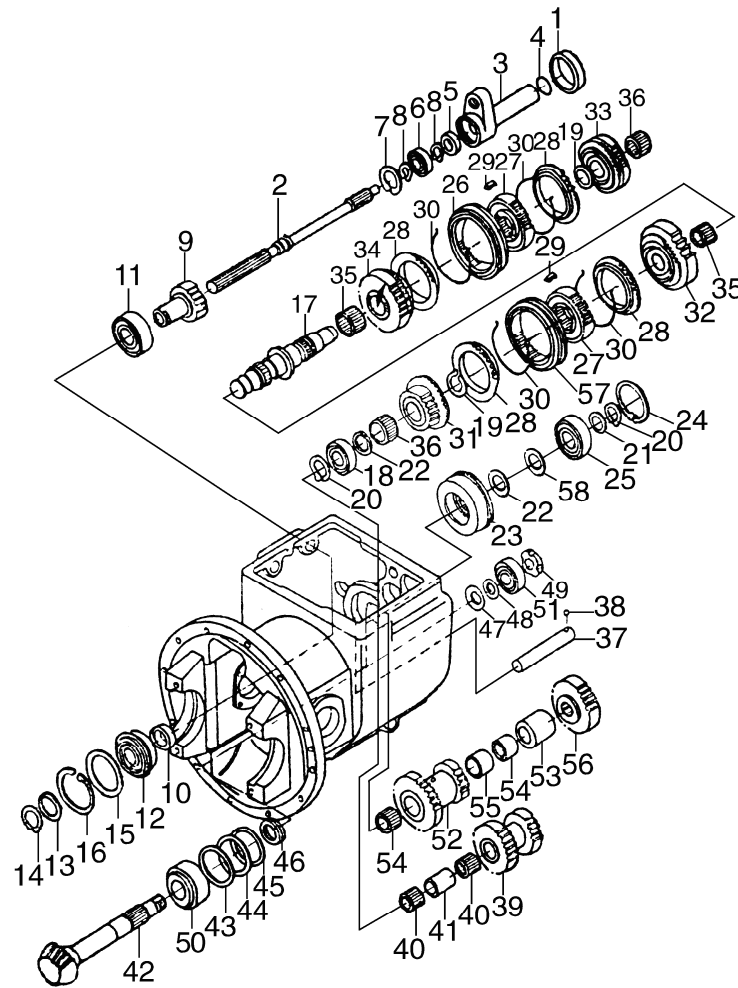
图 16 变速器(机械式 其 2)中南 ZhongNan Fig.16 Transmission(clutch type part-2)
