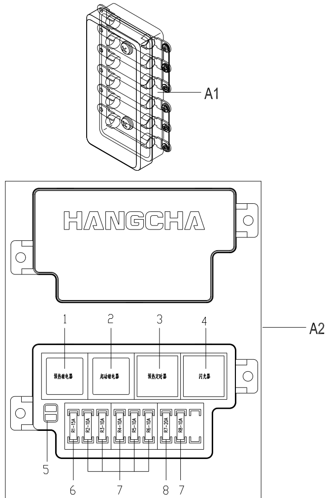
图V 控制盒总成 Fig.V Control box assy
