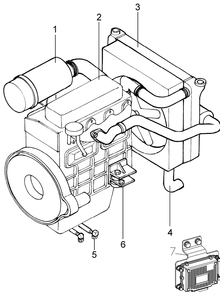
图 1 动力系统 Fig.1 Power system
