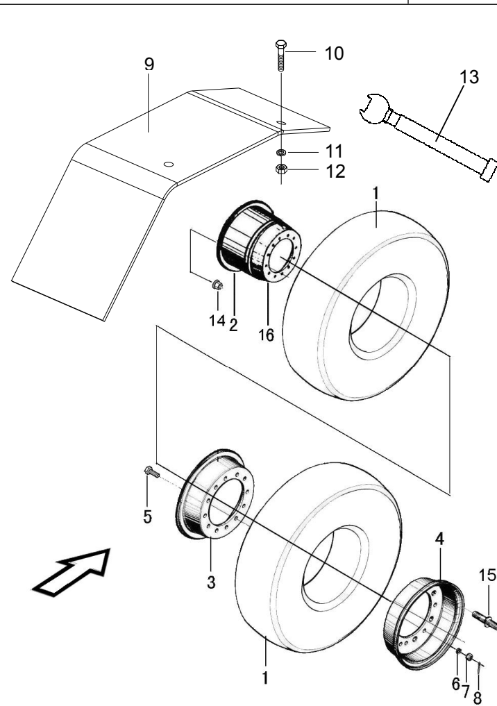
图 5 1.0t-1.8t 前轮（双轮） Fig.5 1.0t-1.8t Front wheel（Double tyre）
