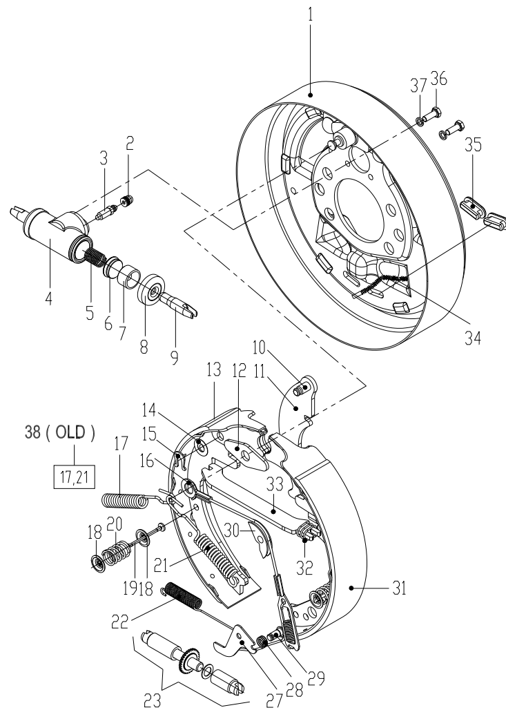
图 7 制动器总成 Fig.7 Brake assy
