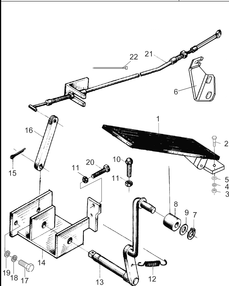
图 5 油门操纵总成 Fig.5 Throttle control assy
